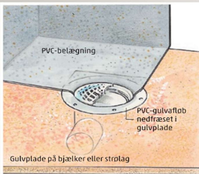
Figur 37 Gulvaflob til PVC-belægning med flange nedfræset i gulvplade før lægning af PVC-belægning. Belægningen føres ned i afløbet og fastgøres med en klemring, der presser belægningen tæt mod afløbet.
