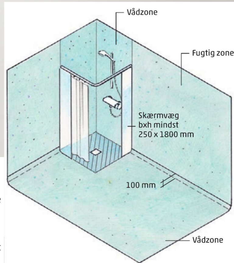
Figur 2 Vådzone og fugtig zone i vådrum med mindst 250 mm brede, fastmonterede skærmvægge omkring bruseniche. Vådzone omfatter hele gulvet og væggene indenfor skærmvæggene. I det skraverede felt bør faldet være mindst 1 % og der må ikke være rørgennemføringer. Vandet skal hindres i at løbe ud af brusenichen, fx ved at forsænke gulvet i nichen.
