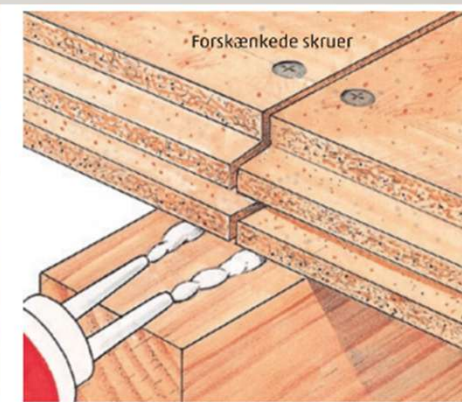
Figur 18 Undergulvsplader limes og skrues altid til bjælker og stroer. Frie kanter skal altid understøttes.
