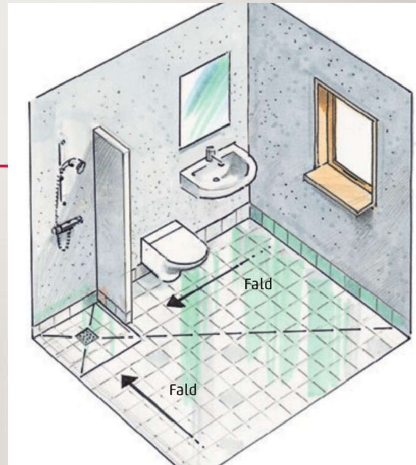
Figur 5 Krav til fald på gulve i vådrum betyder, at gulv i bruseniche bør udføres med et fald på mindst 1 %. Gulvet i den øvrige del af rummet kan udføres med reduceret fald, men der må ikke være bagfald og lunger. Bruseniche udføres bedst med forsænket gulv. Udføres der en opkant foran brusenichen, skal der som regel være et gulvafløb både i brusenichen og ét i rummet i øvrigt.
