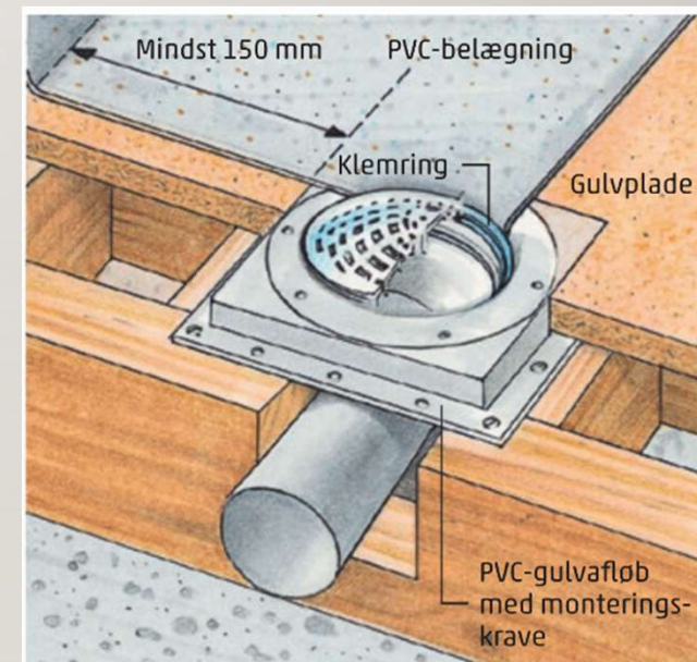
Figur 35 Gulvaflob med krave til PVC-belægning. Gulvaflobet fastgøres til bjælkelag for lægning af godkendte gulvplader. PVC-belægning føres ned i afløbet og tættes med en klemring.
