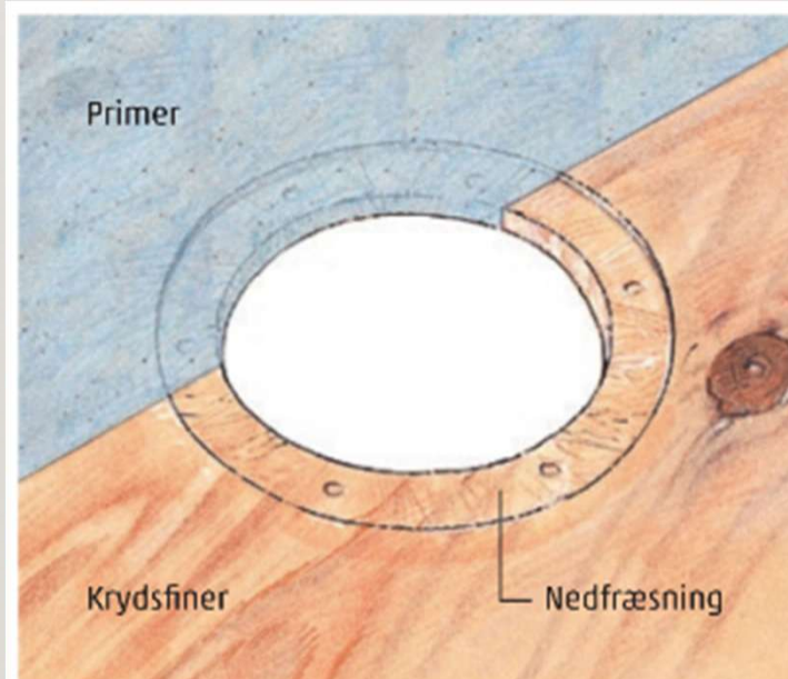
Figur 36 Nedfræsning for gulvaflob udføres, så gulvaflobets flange ligger plant med træpladens overside. Træpladen primes før gulvaflobet monteres, se figur 40.
