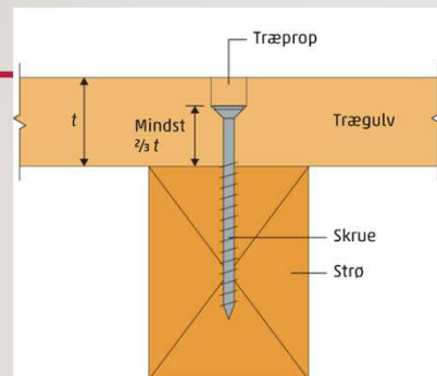
Figur 116 Propning af skruer med afstikning af træprop. Træpropen må højst fylde 1/3 af brættets tykkelse.
