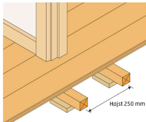
Figur 129 Brædder kan forløbes gennem døråbninger ved døre uden bundstykke, men bør kun udføres mellem to mindre rum af stort set samme størrelse.
