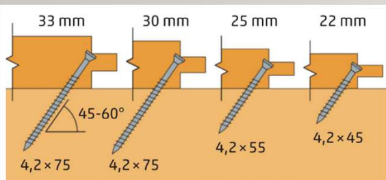
Figur 115 Placering og dimensioner på skruer i feren (fordækt fastgørelse). Dimensionerne gælder for skruer iht. tabel 23. For andre skrue/sømtyper og underlag, se tabel 24 og 25.
