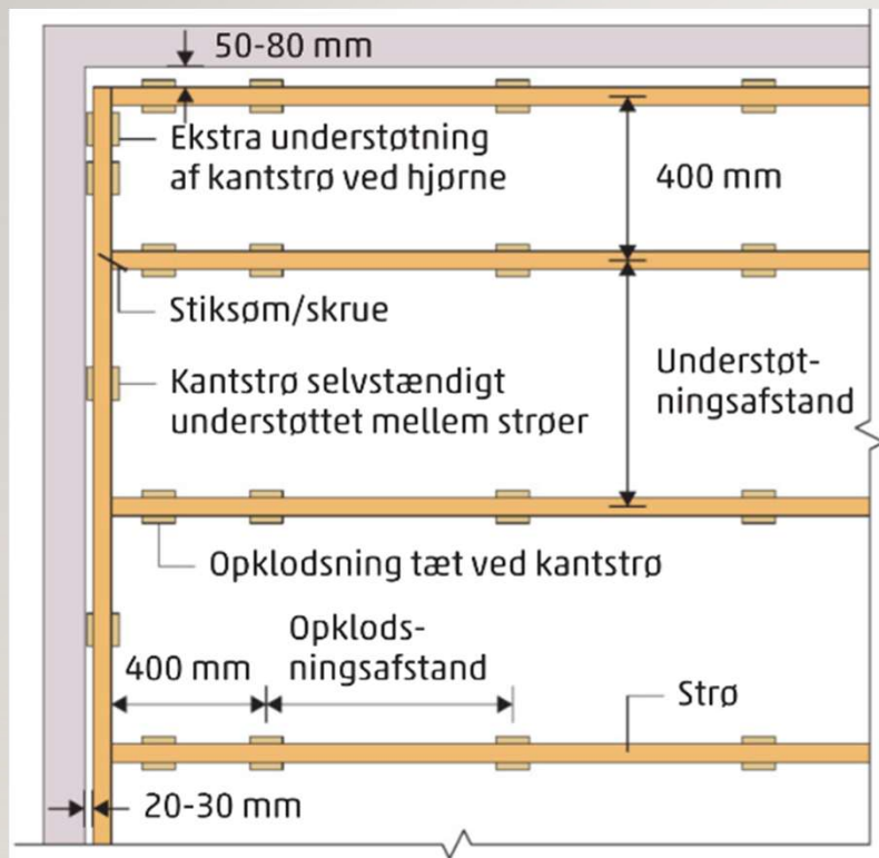
Figur 93 Strølagsmetode 1 med understøtning og fastgørelse af strø og kantstrø langs vægge.
