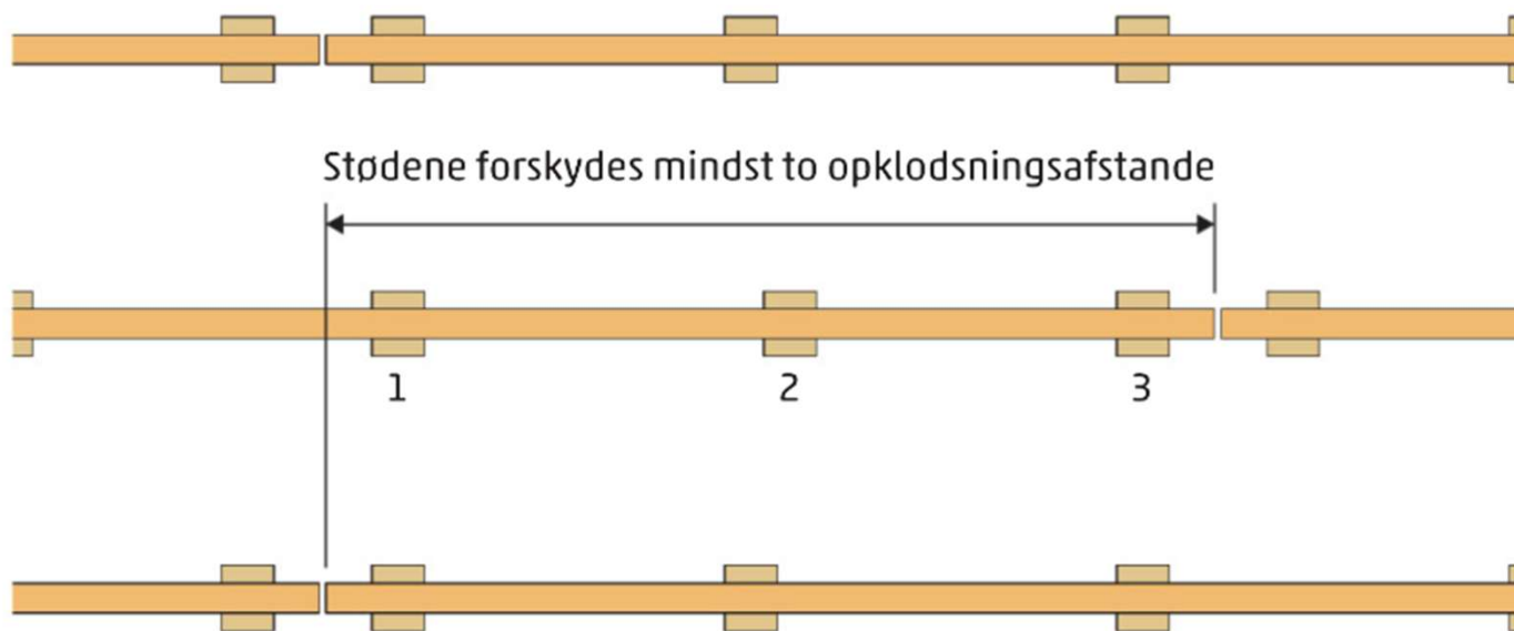
Figur 103 Stød i strøer skal forskydes, så højst hver anden strø er stødt i samme fag. Stødene bør forskydes mindst to opklodningsafstande.
