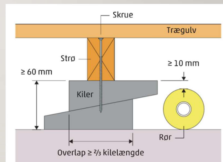
Figur 97 Opklodsning af strøer med træbrikker og evt. bitumenmembran. Er opklodsningen udført på bløde brikker af lydhensyn, må der ikke sømnes i den bløde del af brikken.
