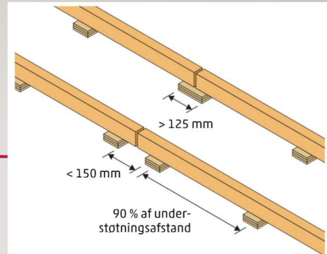
Figur 102 Ved stød i strøer skal begge ender opklodses og opklodningsafstanden reduceres med mindst 10 %.
