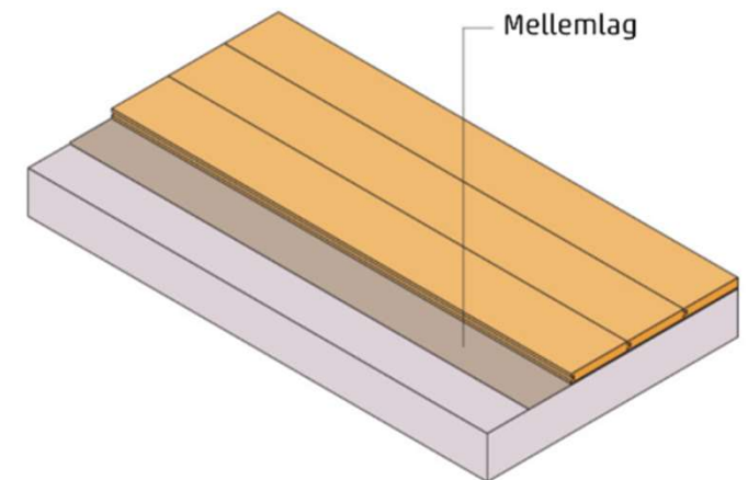
Figur 6 Svømmende, ikke-bærende trægulv.
