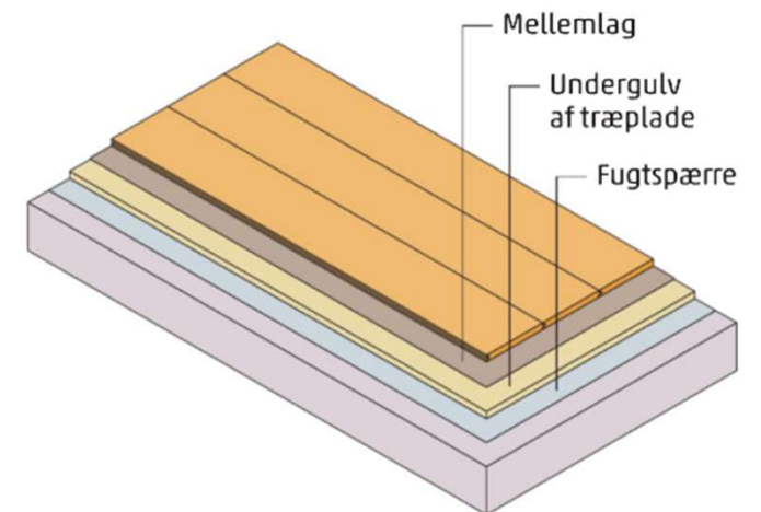
b. Svømmende trægulv på undergulv af træplade på beton
