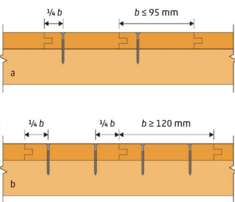
Figur 113 Forsænket fastgørelse med skruer. a. I smalle brædder ca. 1/4 fra brættets notside. b. I brædder bredere end ca. 120 mm med to skruer.
