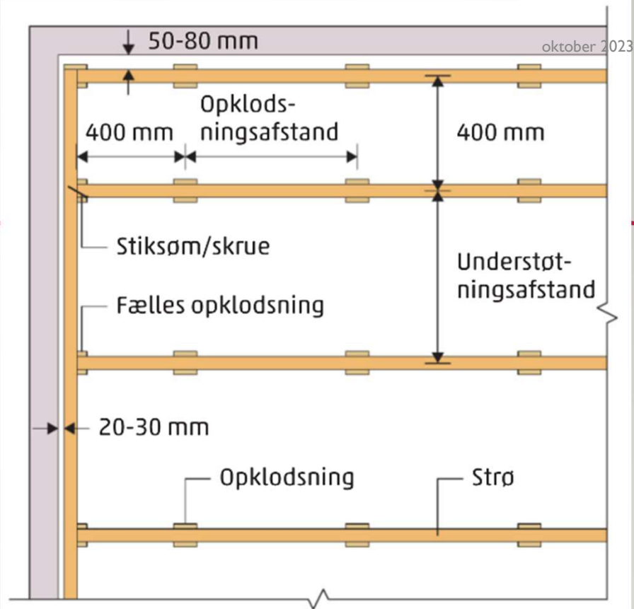
Figur 92 Strølagsmetode 1 med kantstrø: Strølægning med reduceret afstand mellem 1. og 2. strø. Kantstrø fastgøres til gulvstrøerne og opklodses enten på fælles opklodsning ved strøender eller midt imellem strøer, se figur 93. Metoden anvendes også til almindelige undergulve med træplader, fx spånplader, iht. tabel 22 side 144.
