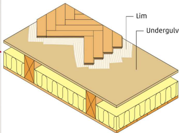
a. Fuldlimet trægulv på træunderlag
