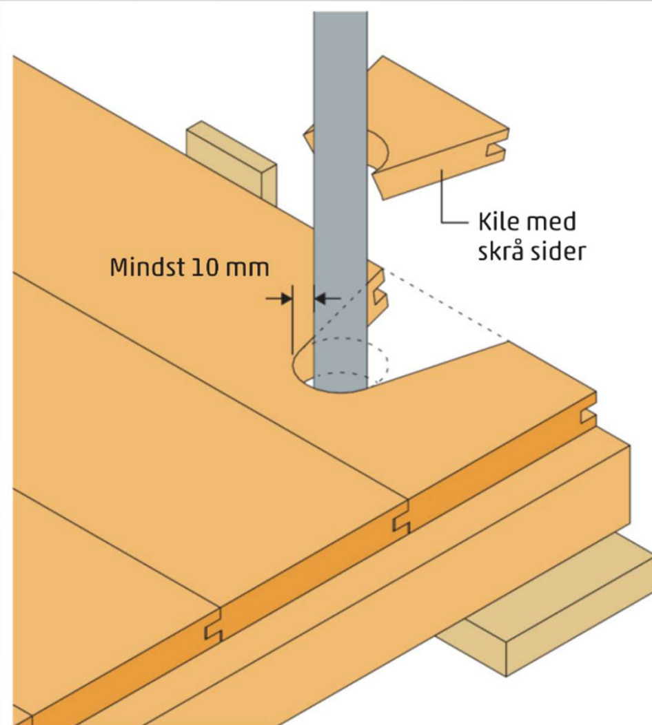
Figur 133 Udsækning for rør. Kilen har skrå sider, så den låser sig selv fast ved limning.
