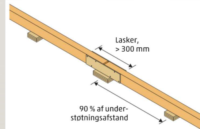
Figur 104 Laskesamling af stød i strø. Stødet skal altid opklodses, og opklodningsafstanden skal reduceres til naboopklodning med 10 %.
