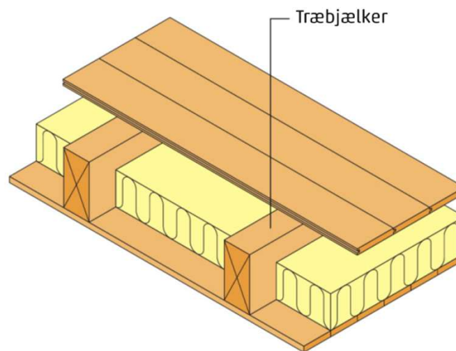
Figur 3 Bærende trægulve på bjælkelag.
