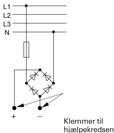
Figur 557.1 – Hjælpeleds forsynet direkte fra hovedkredsen
