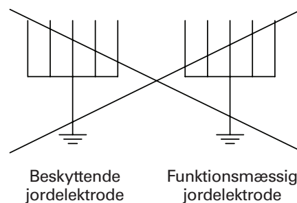
Figur 44.R11 – Indbyrdes forbundne jordelektroder
