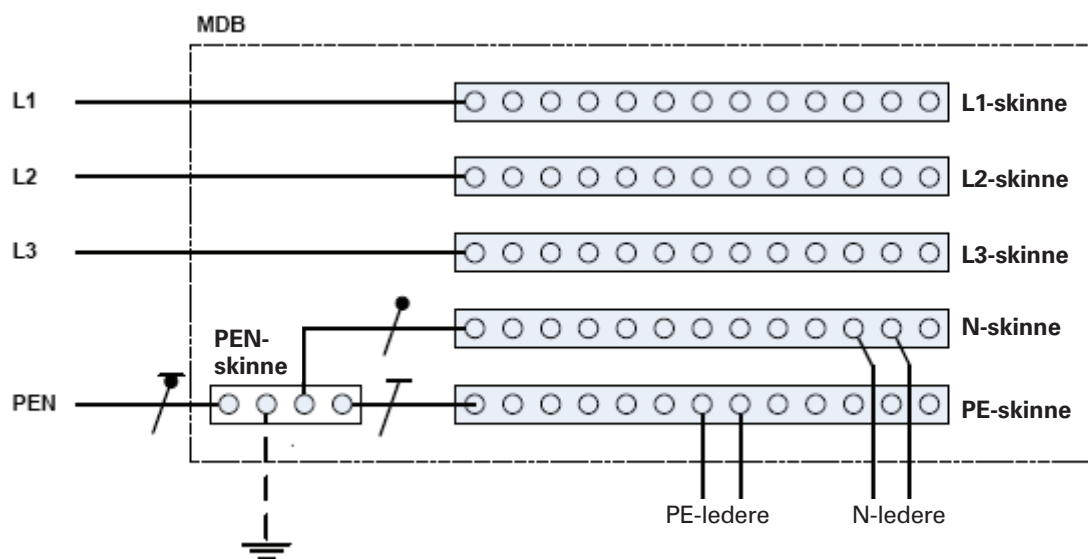
Figur 54.1c – Eksempel 3
