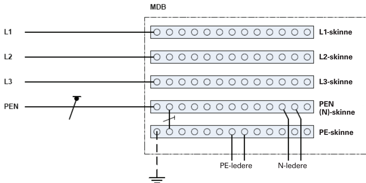
Figur 54.1b – Eksempel 2
