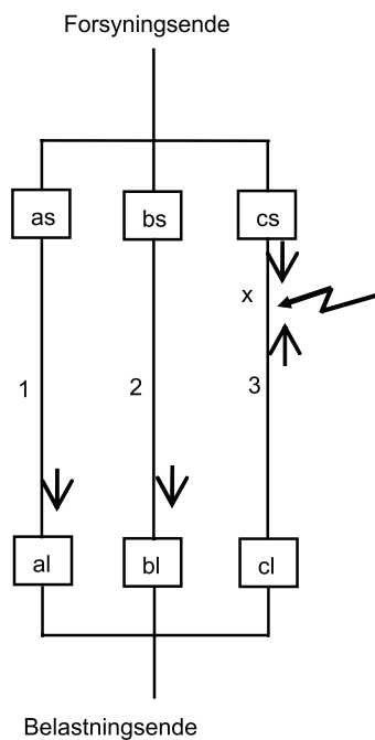
Figur A.3 – Strømforløb ved fejlens opståen
