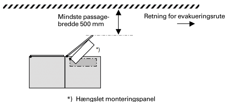
Figur 729 A.2 – Mindste passagebredde i forbindelse med evakuering –Tilfælde 2
