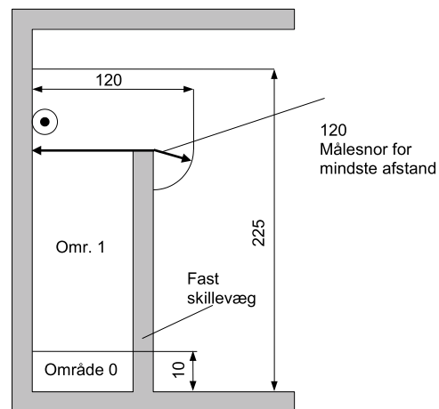
2) Set fra siden (med fast skillevæg og radius for mindste afstand over skillevæggen)
