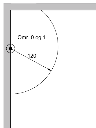
2) Set fra siden (med fast skillevæg og radius for mindste afstand over skillevæggen)
