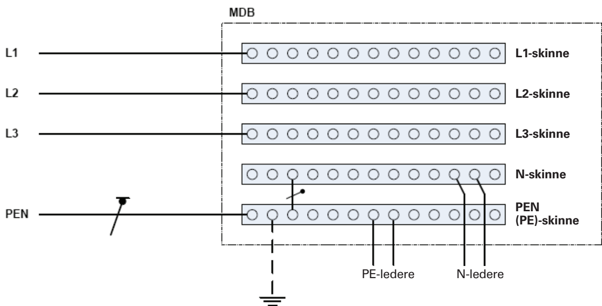
Figur 54.1a – Eksempel 1
