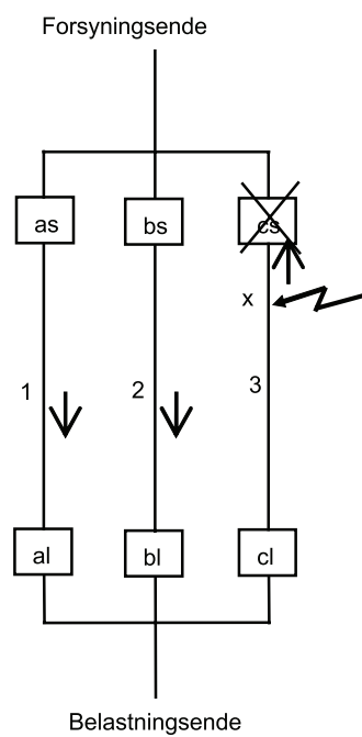
Figur A.4 – Strømforløb efter udløsning af beskyttelsesudstyret cs
