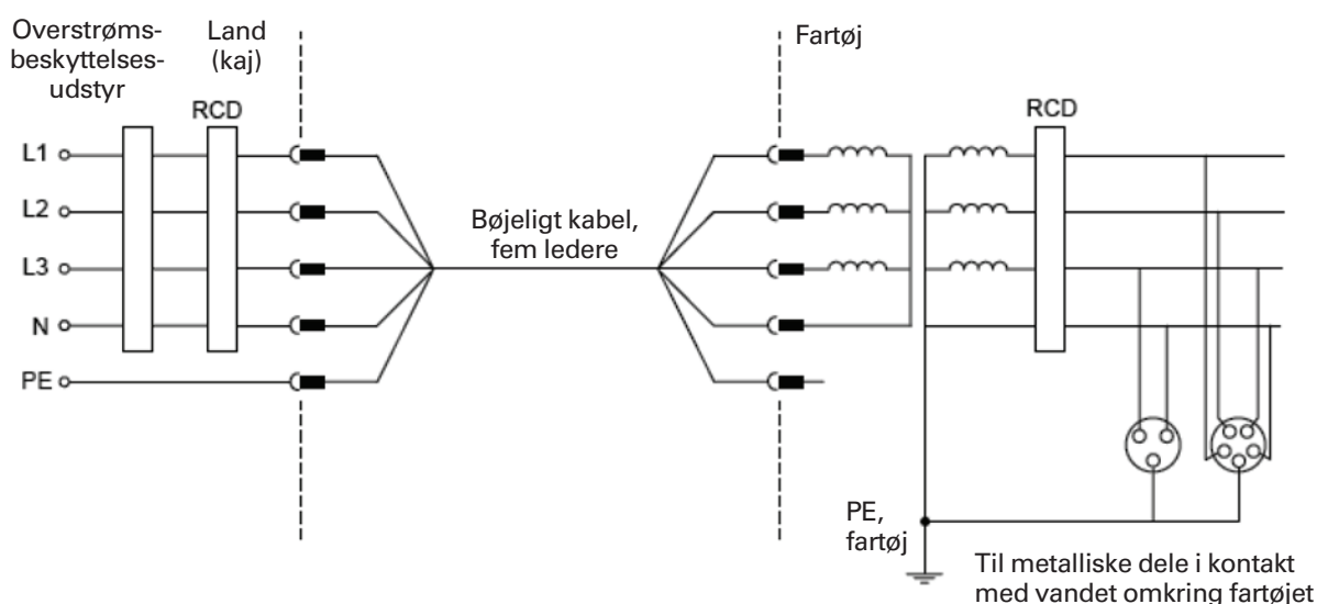
Figur 730A.3 – Direkte forbindelse til en trefaset netforsyning
