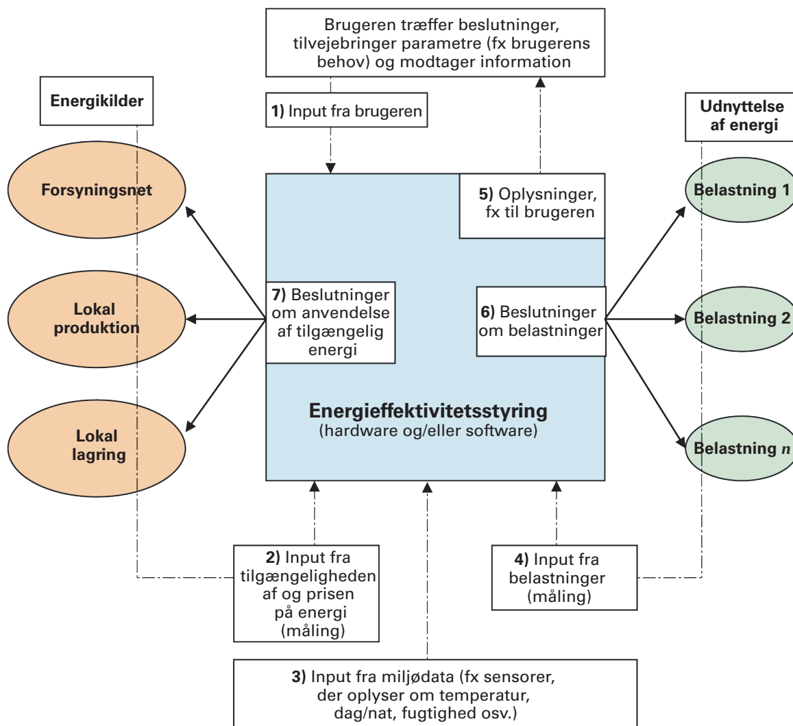
Figur 1 – Energiefektivitets- og belastningsstyringssystem, oversigt
