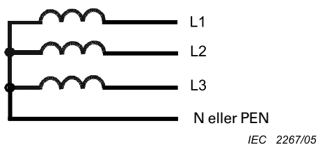
Figur 5 – Trefaset 4-leder
