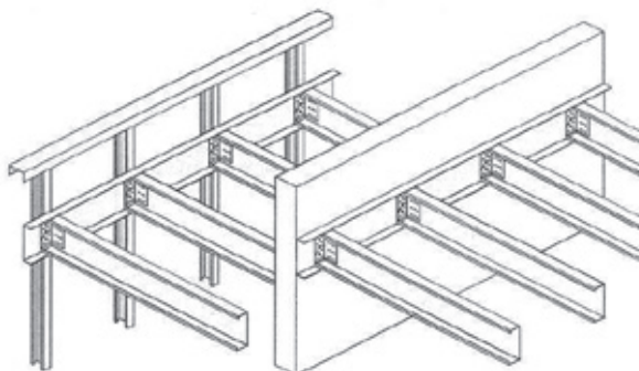
Etagedæk monteret på siden af bærende væg.
