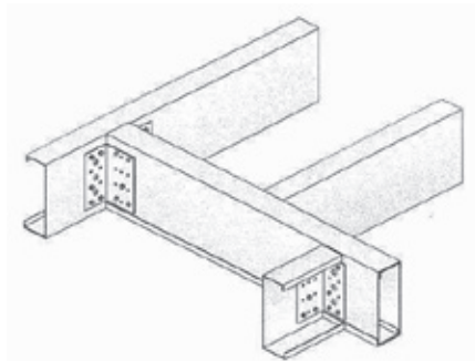
Brug evt. dobbelt C-profil, hvis udvekslingsprofilerne skal bære C-profiler i begge retninger.
