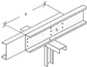
Samling af C-profiler over bærende indervæg.
