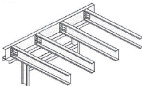
Etagedæk monteret ovenpå bærende væg.
