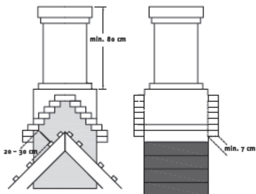
Traditionel udkravet skorsten.
