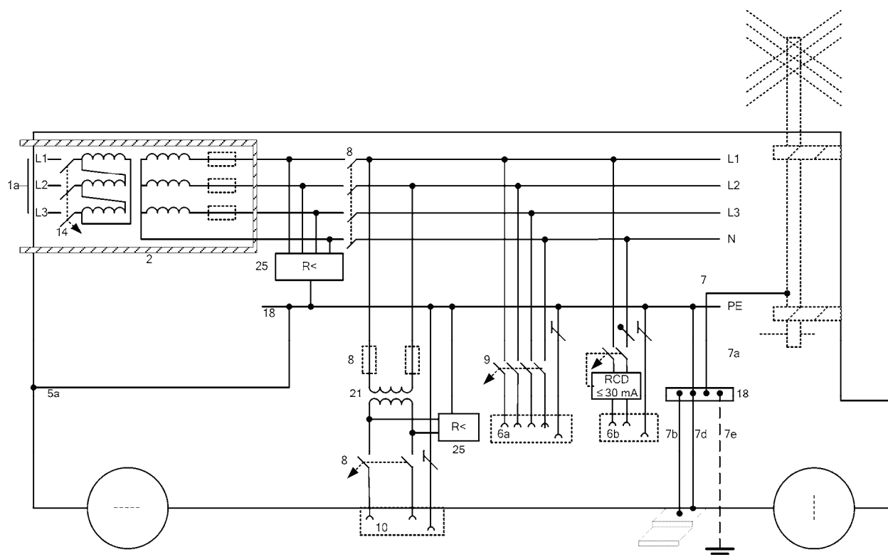
Figur 717.7 – Eksempel på forbindelse til en fast elektrisk installation med en vilkårlig type jordningssystem ved hjælp af et IT-system uden automatisk afbrydelse ved første fejl
