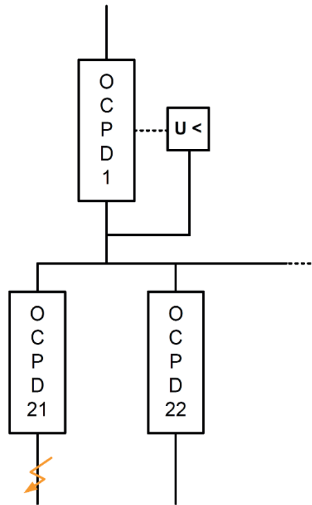
Figur 536.11 — Selektivitet mellem OCPD og underspændingsrelæer
