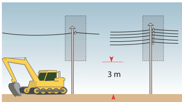
Højspændingsluftledning 10-40 kV
