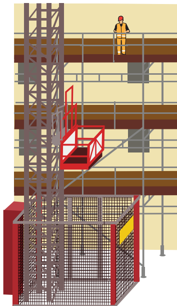
Materialehejs
