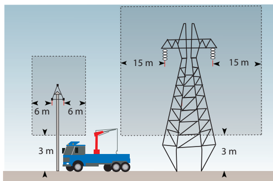
Højspændingsluftledning 10-40 kV
