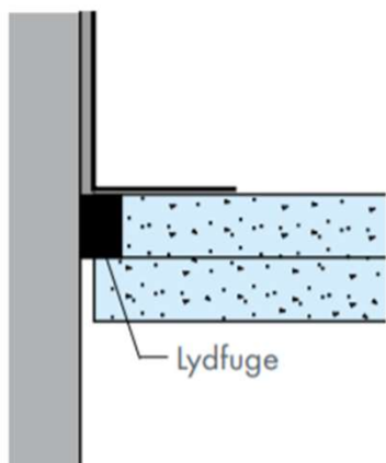
Lydfuger ved flankerende vægge af andre materialer end gips.
