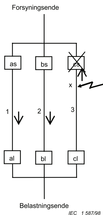
Figur A.4 – Strømforsyning og fejlstrøm i en parallel leder efter udløsning af beskyttelsesudstyret cs
