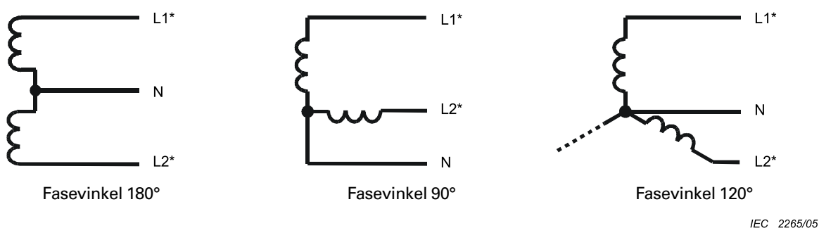
Figur 2 – Enfaset 3-leder
