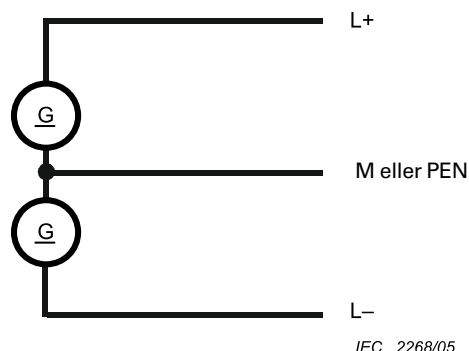
Figur 7 – 3-leder
