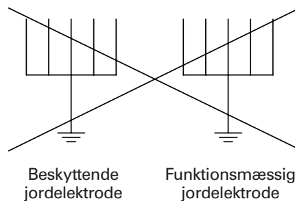
Figur 44.R11 – Indbyrdes forbundne jordelektroder
