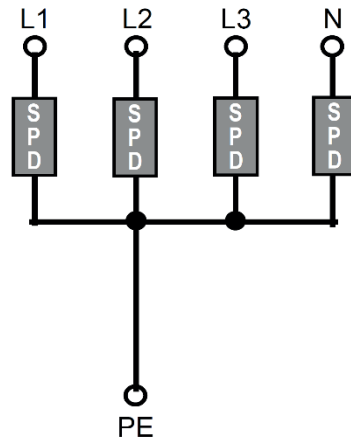
Figur 534.2 — Forbindelsestype CT1 (4+0-konfiguration) for et trefasesystem med nulleder
