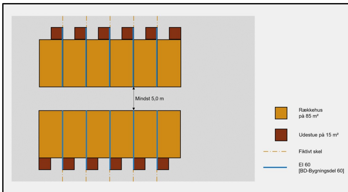
Figur 1.3.5 Eksempel på rækkehusbebyggelse i brandmæssigt fritliggende bygningsafsnit på 510 m² med ligelig mulighed for tilbygning.
