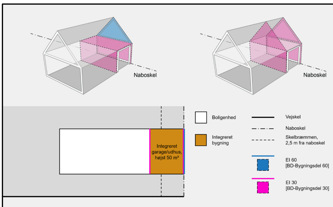
Figur 4.13.3 Integreret garage/udhus på højst 50 m 2 , adskilt fra boligenheden og mod naboskel med bygningsdel EI 30 [BD-bygningsdel 30]. Hvis adskillelsen etableres i etageadskillelsen skal tagkonstruktionen adskilles mod skel med bygningsdel (R)EI 60 [BD-bygningsdel 60].
