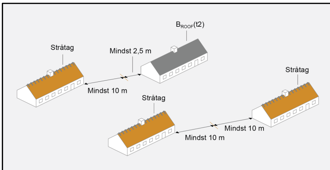
Figur 4.2.2 Afstanden mellem enfamiliehuse på samme grund, hvis et eller flere af bygningerne har tagdækning, som ikke er tagdækning klasse B_{ROOF}(t2) , og stråtagene ikke er brandsikret.
