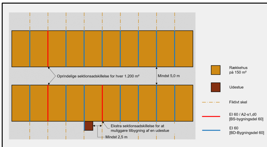
Figur 1.3.6 Eksempel på rækkehusbebyggelser på 1.500 m² opdelt i bygningsafsnit på højst 1.200 m².
