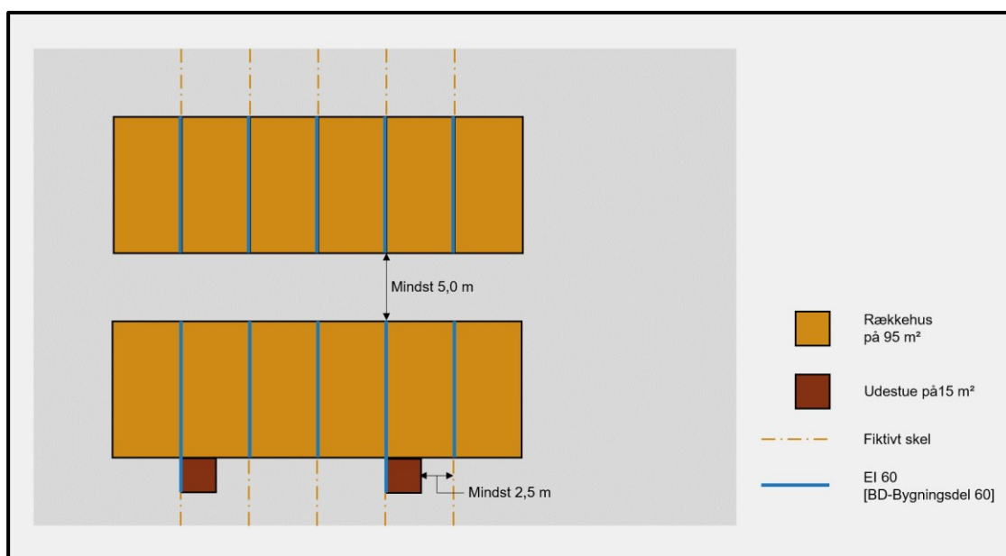
Figur 1.3.4 Eksempel på rækkehusbebyggelse i brandmæssigt fritliggende bygningsafsnit på 570 m² med begrænset mulighed for tilbygning.
