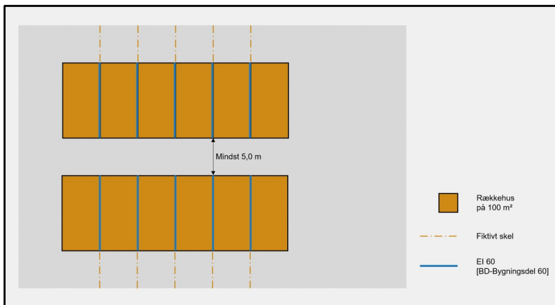
Figur 1.3.3 Eksempel på rækkehusbebyggelse i brandmæssigt fritliggende bygningsafsnit på 600 m².
