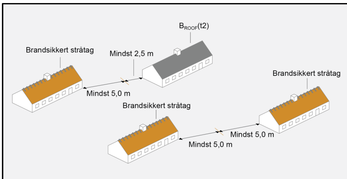
Figur 4.2.1 Afstanden mellem enfamiliehuse på samme grund, hvis et eller flere af bygninger har tagdækning, som ikke er tagdækning klasse B_{ROOF}(t2) , men hvor stråtagene er brandsikret.
