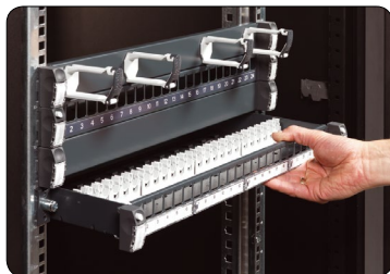
8. Patchpanelet trækkes ud til stoppet og der kan nu monteres konnektorer og kabler.
