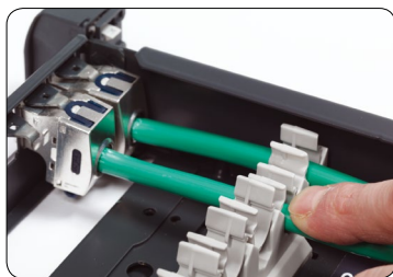
12. Kablerne trykkes i kabelorganisatoren og derved undgås strips.
