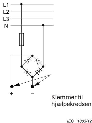
Figur 557.2 – Hjælpeleds forsynet via ensretter fra hovedkredsen
