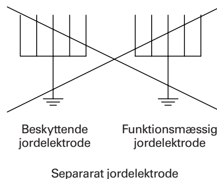
Figur 44.R11 – Indbyrdes forbundne jordelektroder
