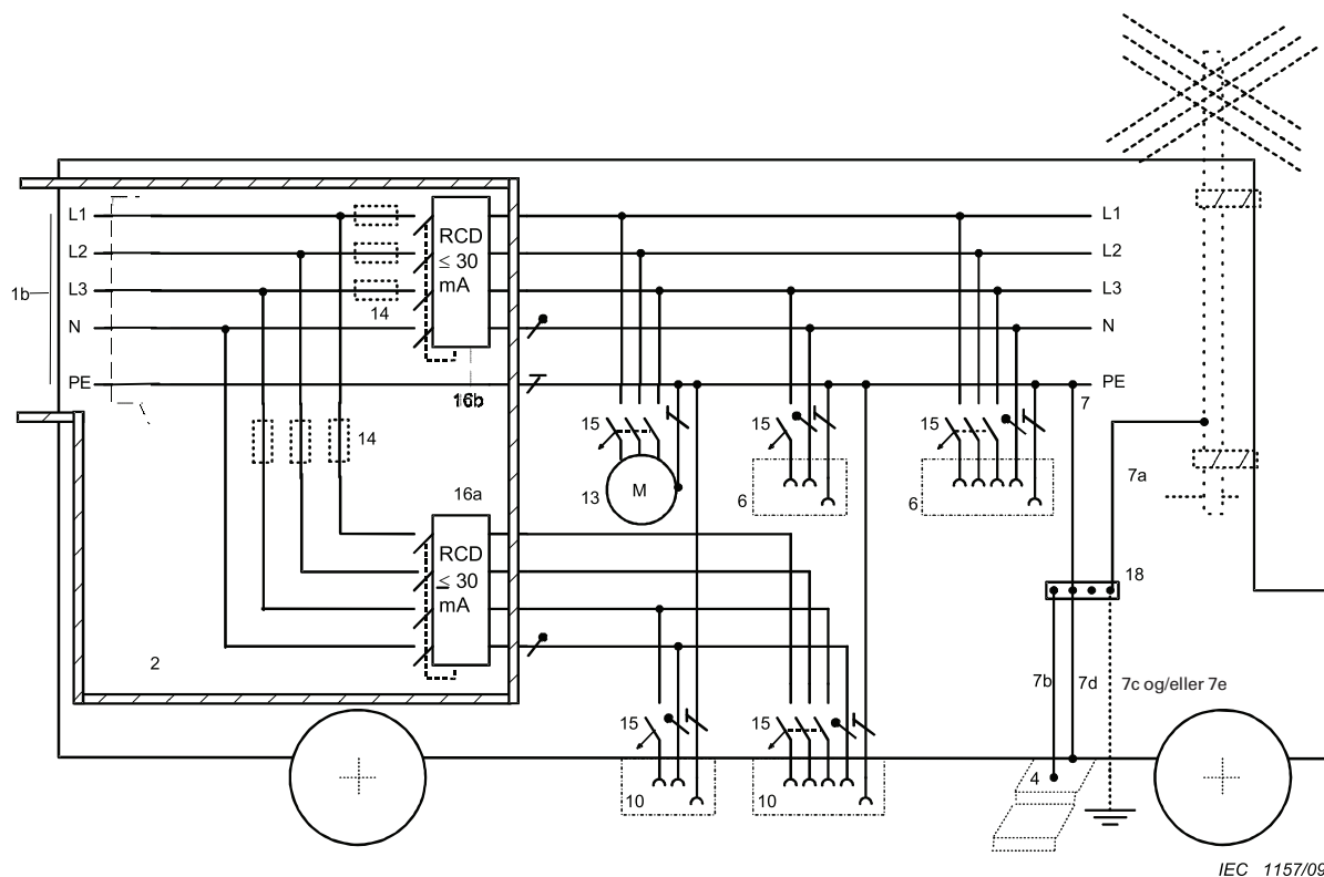
Figur 717.3 – Eksempel på forbindelse til enhver type jordingssystem i en fast installation med automatisk afbrydelse af forsyningen ved hjælp af RCD (fejlstrømsafbrydere), med eller uden jordelektrode
