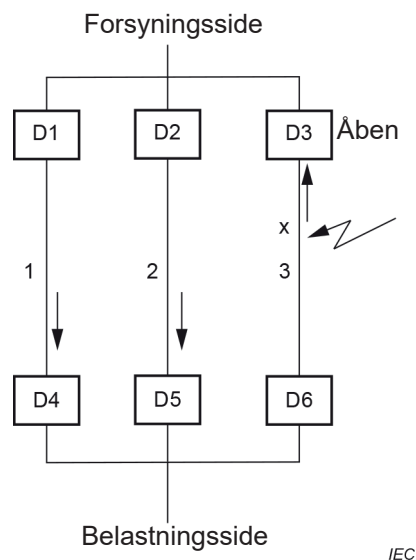
Figur C.3 – Strømforløb ved kortslutningens begyndelse
