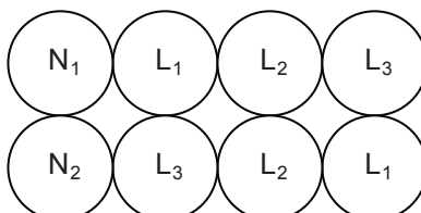
Figur H.52.2 – Særlig konfiguration for 6 parallelle enlederkabler over hinanden (se 523.7)
