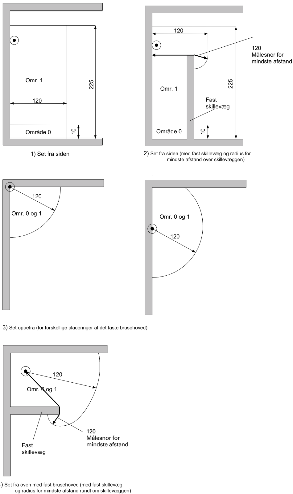
Figur 701.2 – Mål for områderne 0 og 1 i rum med bruser uden bassin
