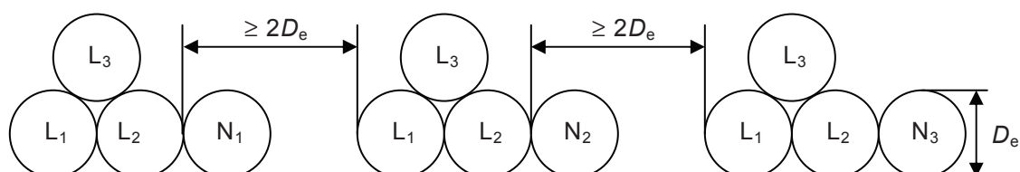
Figur H.52.6 – Særlig konfiguration for 9 parallelle enlederkabler i trekant (se 523.7)
