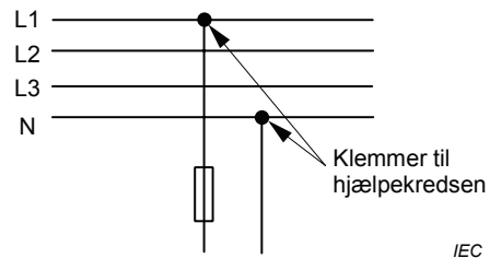
Figur 557.1 – Hjælpeleds forsynet direkte fra hovedkredsen
