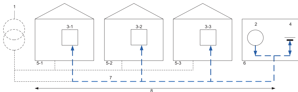
Figur B.6 – Eksempel på elektrisk design af kollektiv PEI, der betjenes i ødriftstilstand med en samlet elinstallation
