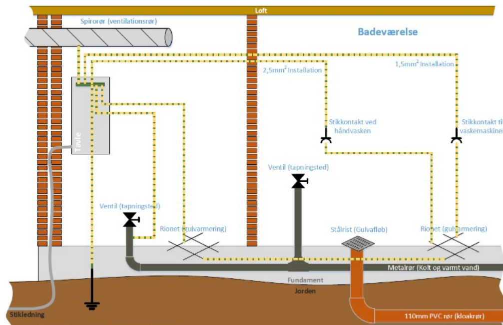
Snittegning
