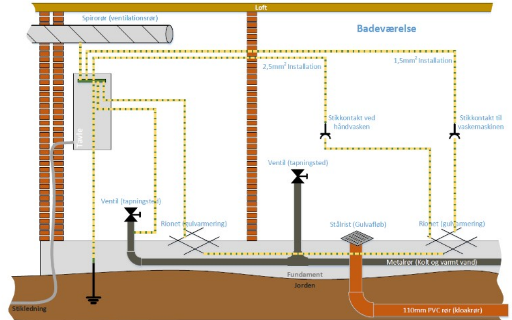
Snittegning
