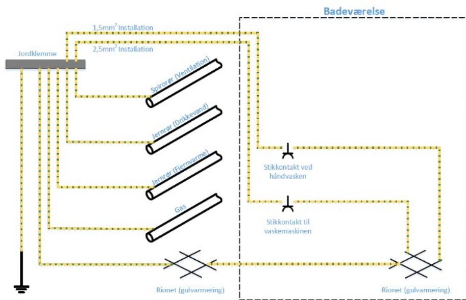
Principtegning
