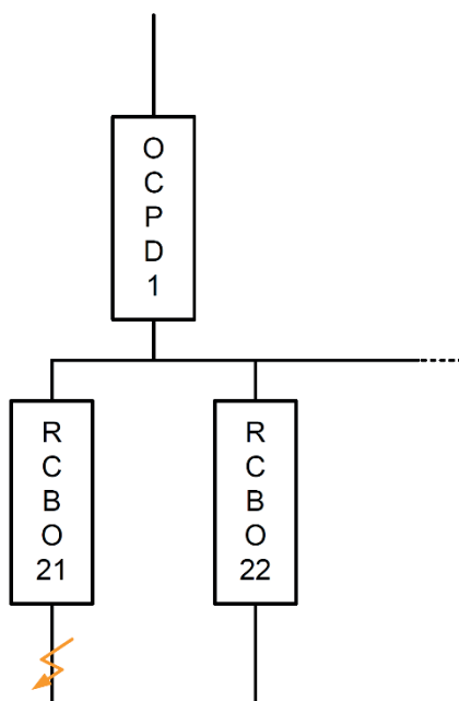
Figur 536.3 — Selektivitet mellem OCPD og RCD ved anvendelse af RCBO'er
