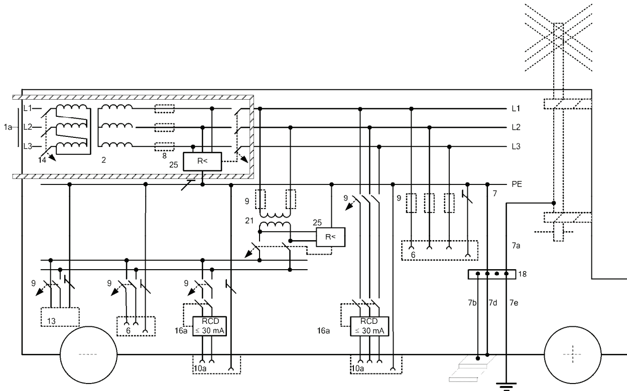
Figur 717.5 – Eksempel på forbindelse med separat strømkreds og et IT-system med isolationsovervågningsudstyr og afbrydelse af forsyningen efter en første fejl
