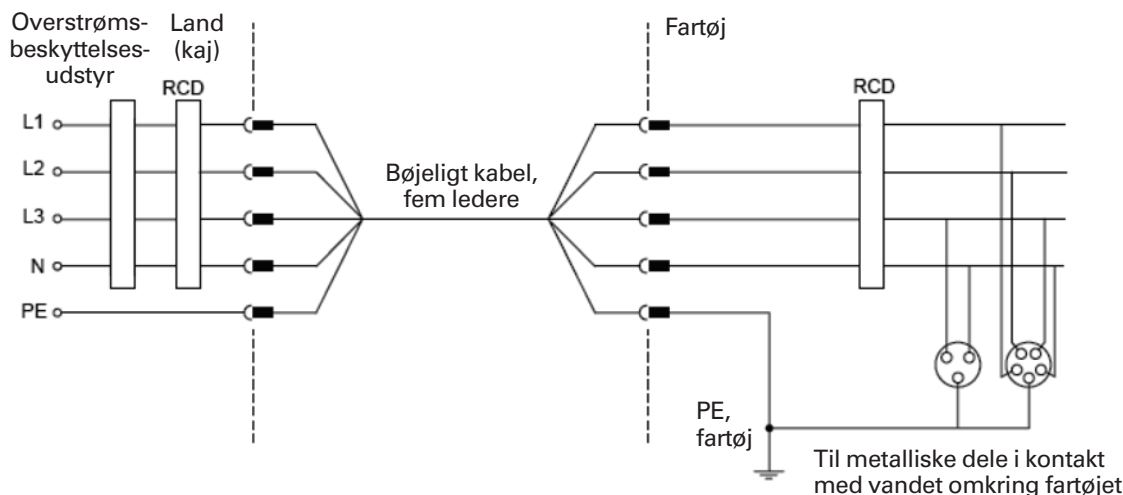
Figur 730A.3 – Direkte forbindelse til en trefaset netforsyning
