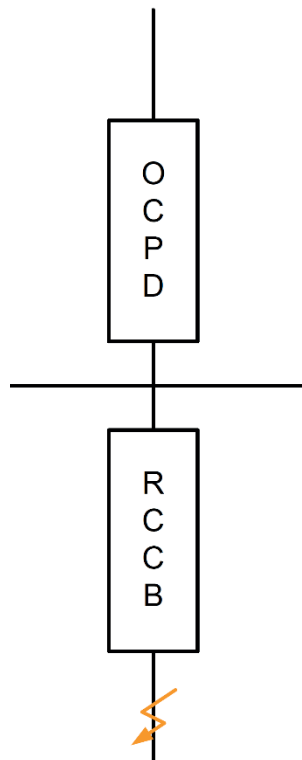
Figur 536.10 — Koordinering af OCPD og RCCB
