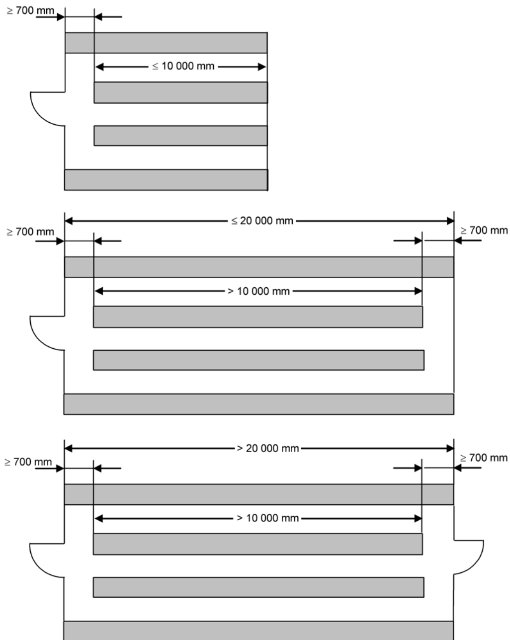
Figur 729.5 – Eksempler på placering af døre i lange, lukkede områder med begrænset adgang
