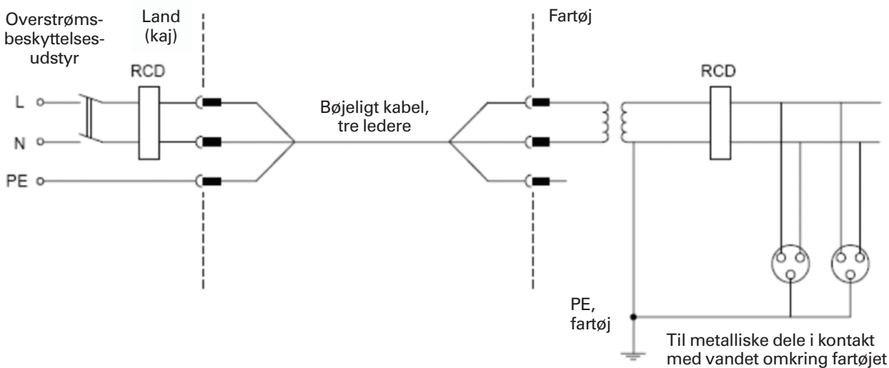
Figur 730A.1 – Direkte forbindelse til en enfaset netforsyning
