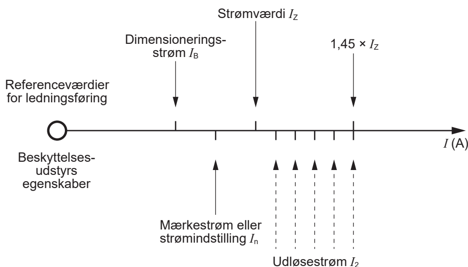
Figur 1 – Koordinering mellem leder og beskyttelsesudstyr (betingelse 1 og 2)
