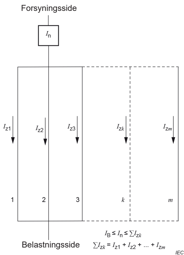
Figur C.2 – Strømkreds med et enkelt overbelastningsbeskyttelsesudstyr i de m parallelforbundne ledere
