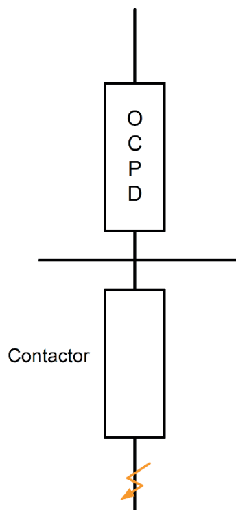
Figur 536.7 — Koordinering af OCPD og kontaktor i tilfælde af kortslutning
