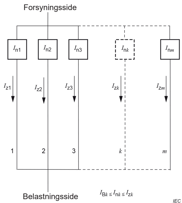
Figur C.1 – Strømkreds med overbelastningsbeskyttelsesudstyr i hver af de m parallelforbundne ledere
