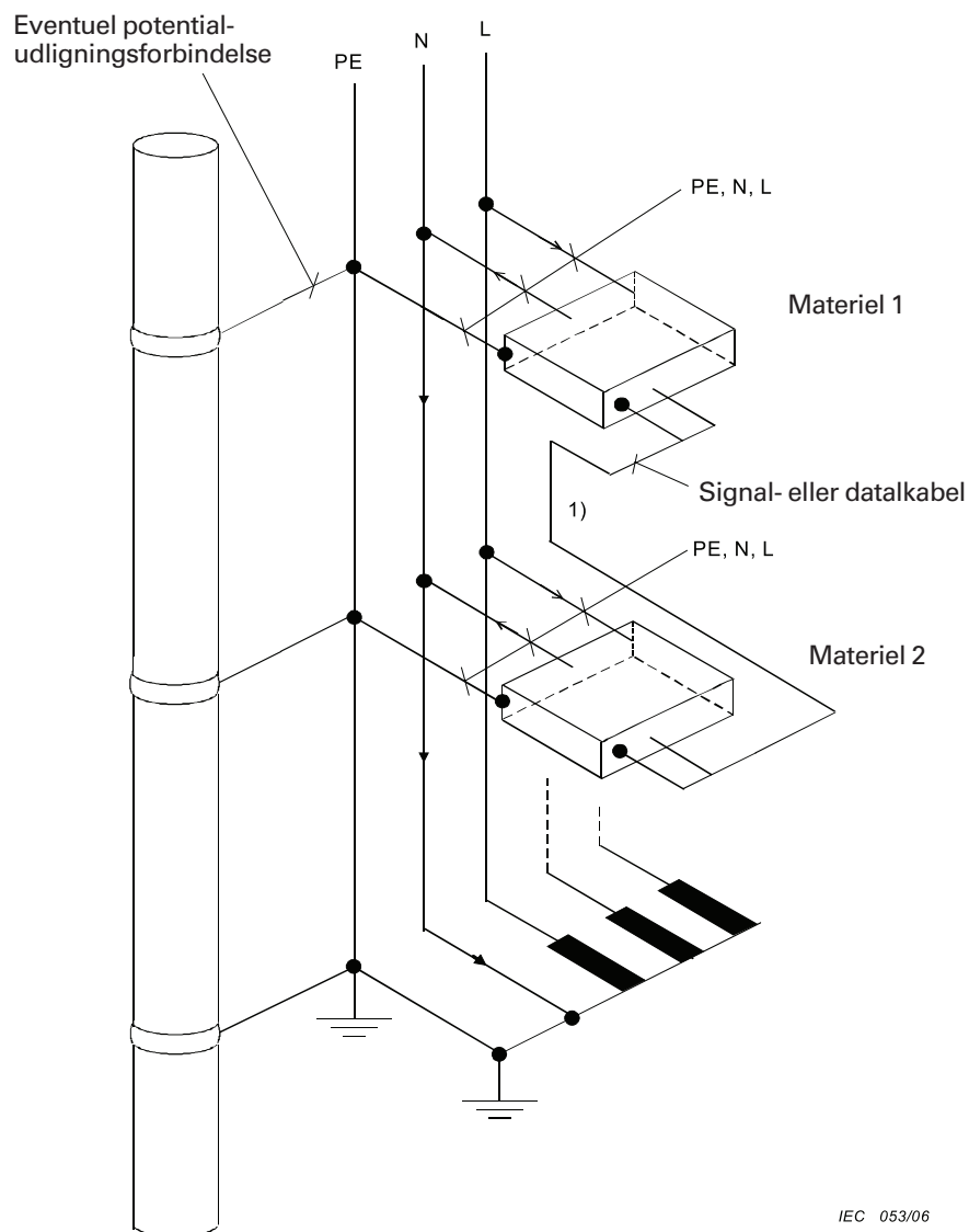
Figur 44.R3B – Eliminering af nullederstrømme i en udlignet struktur ved anvendelse af TN-S-system downstream fra en forbrugers egen forsyningstransformer
