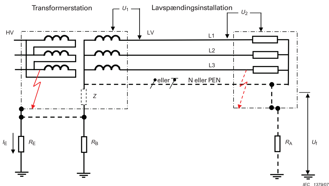
Figur 44.A1 – Repræsentativ skematisk tegning for mulige forbindelser til jord i transformerstation og lavspændingsinstallation og opstående overspændinger i forbindelse med fejl
