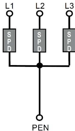
Figur 534.3 — Forbindelsestype CT1 (3+0-konfiguration) for et trefasesystem
