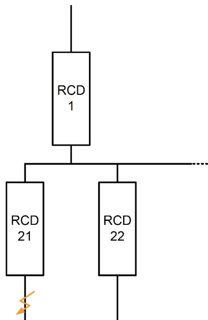
Figur 536.2 — Selektivitet mellem RCD'er i tilfælde af reststrøm
