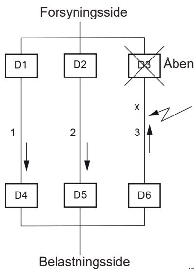
Figur C.4 – Strømforløb efter aktivering af beskyttelsesudstyr D3
