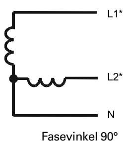
Figur 2 – Enfaset 3-leder
