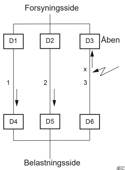
Figur C.3 – Strømforløb ved kortslutningens begyndelse
