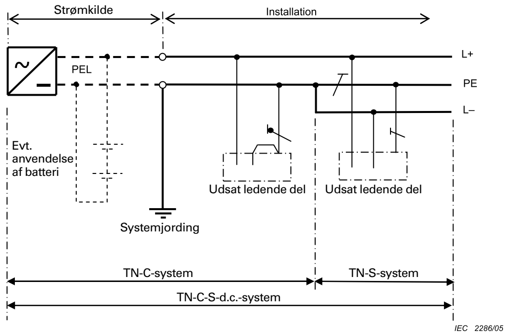
Figur 31K1 – TN-C-S-d.c.-system
