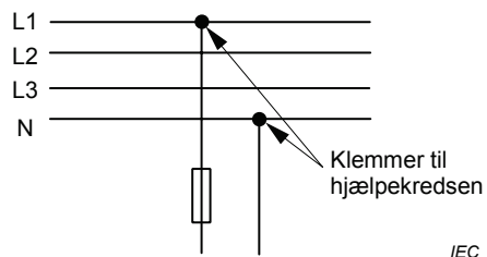
Figur 557.1 – Hjælpeledning forsynet direkte fra hovedkredsen
