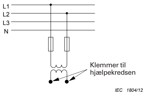
Figur 557.3 – Hjælpeledning forsynet fra hovedkredsen via transformer
