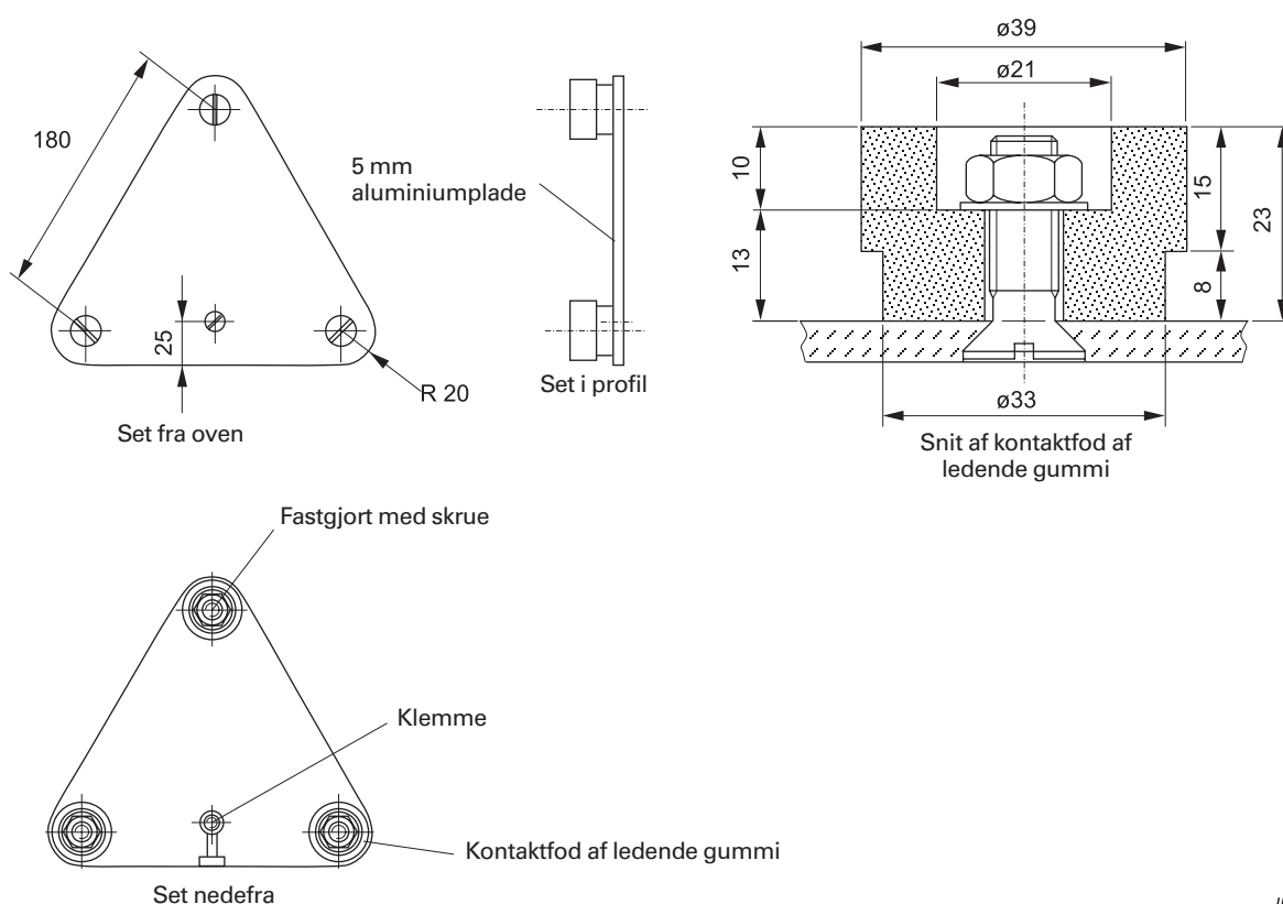
Figur B.1 – Måleelektrode 1
