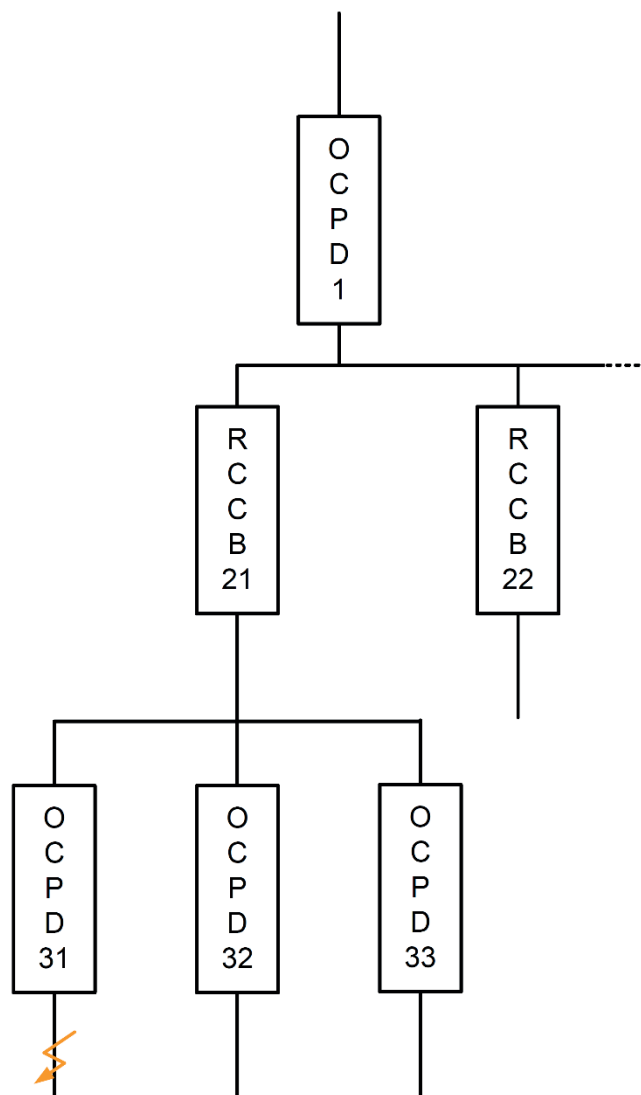
Figur 536.4 — Selektivitet mellem OCPD og RCD ved anvendelse af RCCB'er
