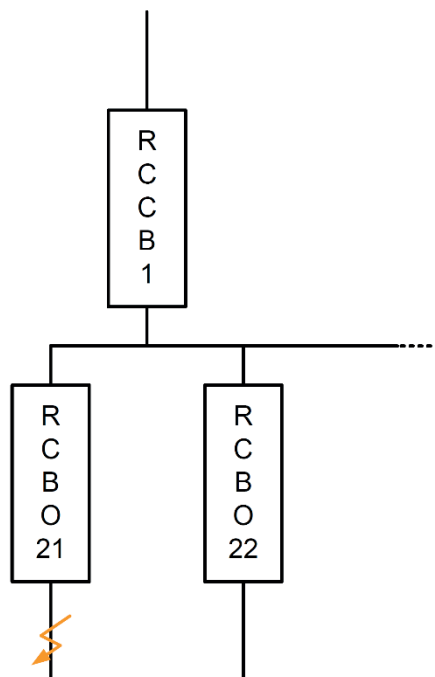
Figur 536.5 — Selektivitet mellem RCCB'en upstream og RCBO'er
