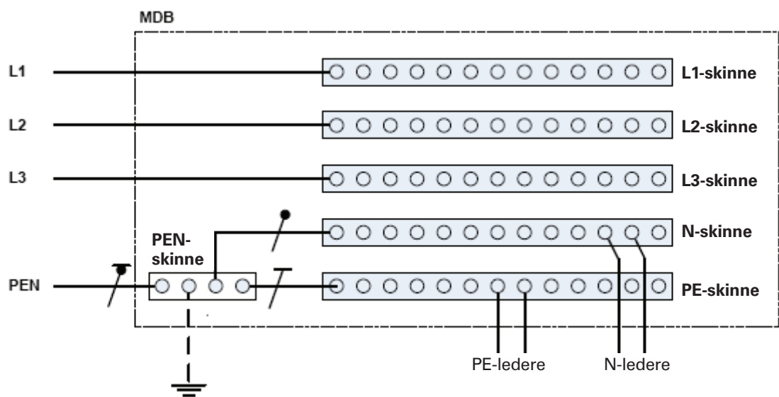
Figur 54.1c – Eksempel 3
