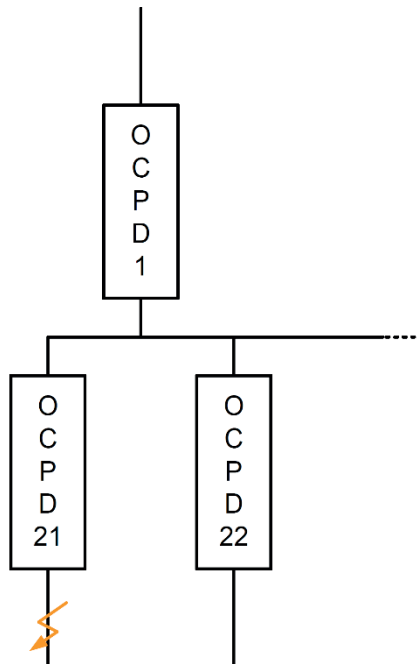
Figur 536.1 — Selektivitet mellem OCPD'er
