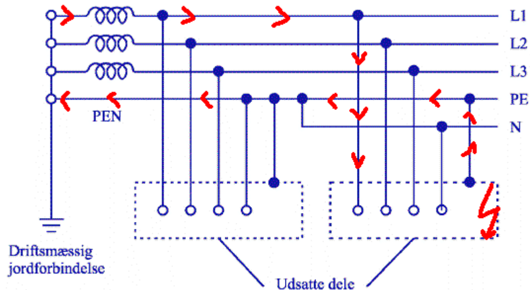
Figur 2 TN-C-S system Nullleder og beskyttelsesleder kombineret i en leder i en del af systemet
