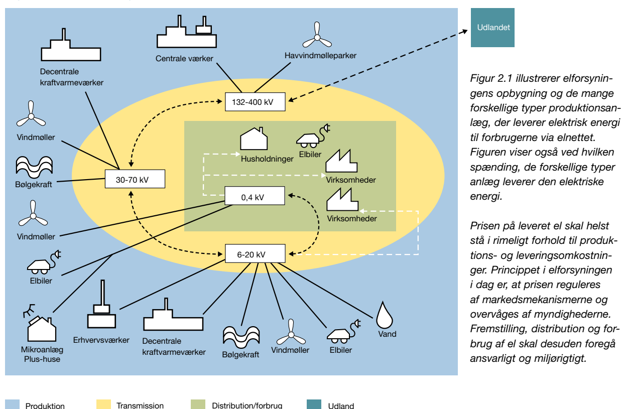
Figur 2.1: Elforsyning i Danmark
