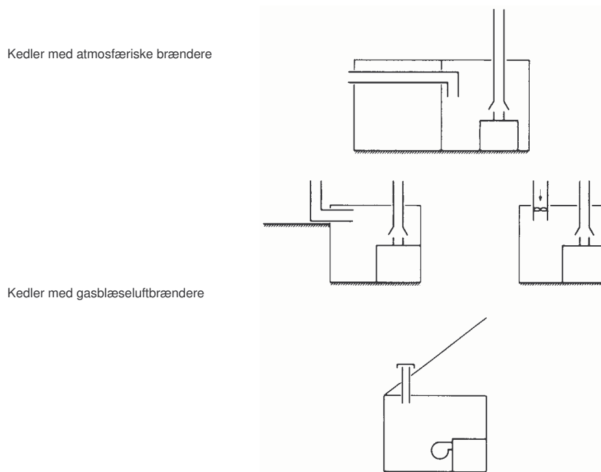
Fig. 4-4: Eksempler på frisklufttilførsel fremført i kanal
