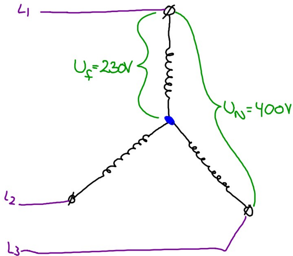
"STJERNE" (Y)
