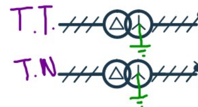
En-streg-tegninger
