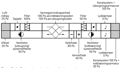
Figur 8.1. Optimale tryktab i ventilationsanlæg.
