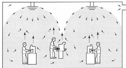
Figur 6.8. Opblandningsprincippet.
