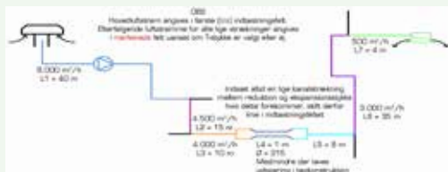
Figur 7.6. Indblæsningskanalstrækning.
