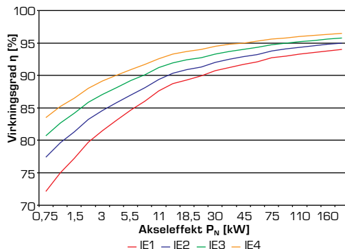
Figur 7.20. Virkningsgrader for 2-polede motorer i henhold til IEC 60034-30:2008 og IEC 60034-31:2010.
